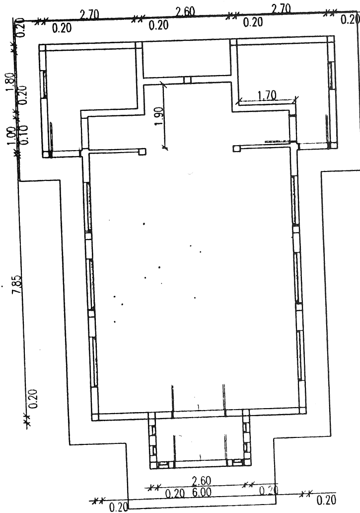
PLANTA ACOTADA
